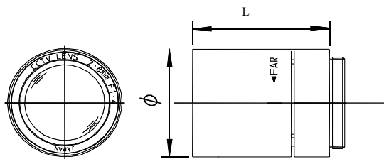
Fixed iris - Manual iris
